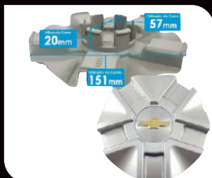
ASTRA SPORT CÓD. 3437A - 6 GARRAS 3,5cm CÓD. 3437B - 6 GARRAS 2cm CÓD. 3437S - 5 GARRAS
